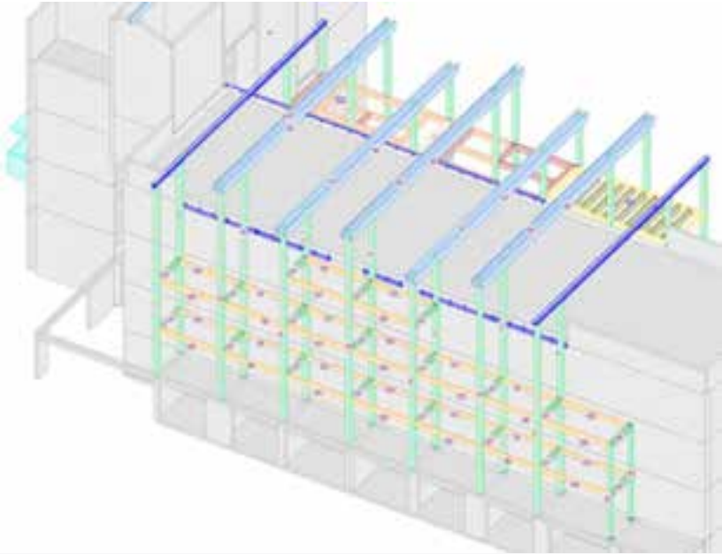
Structure porteuse du bâtiment A – vue façade sud-ouest (balcons) © Toitures Montiliennes
