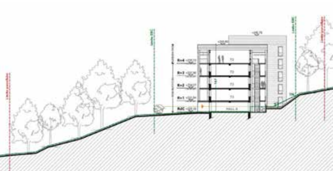
© Adminima architecture / Rhône Saône Habitat - Coupe transversale sur le bâtiment A
