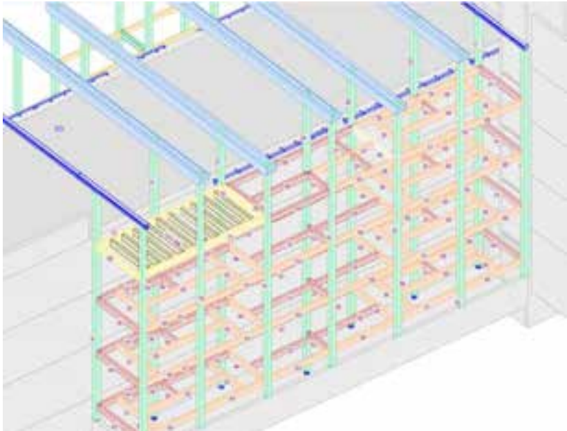
Structure porteuse du bâtiment A – vue façade nord-est (coursives) © Toitures Montiliennes
