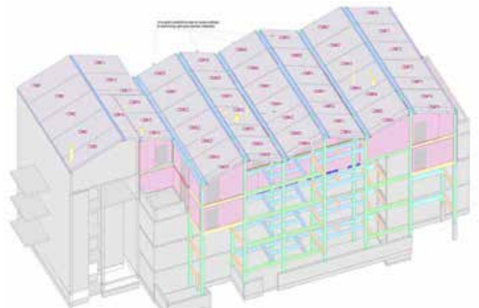
Surélévation du bâtiment B d'un niveau – caissons de toiture préfabriqués © Toitures Montiliennes
