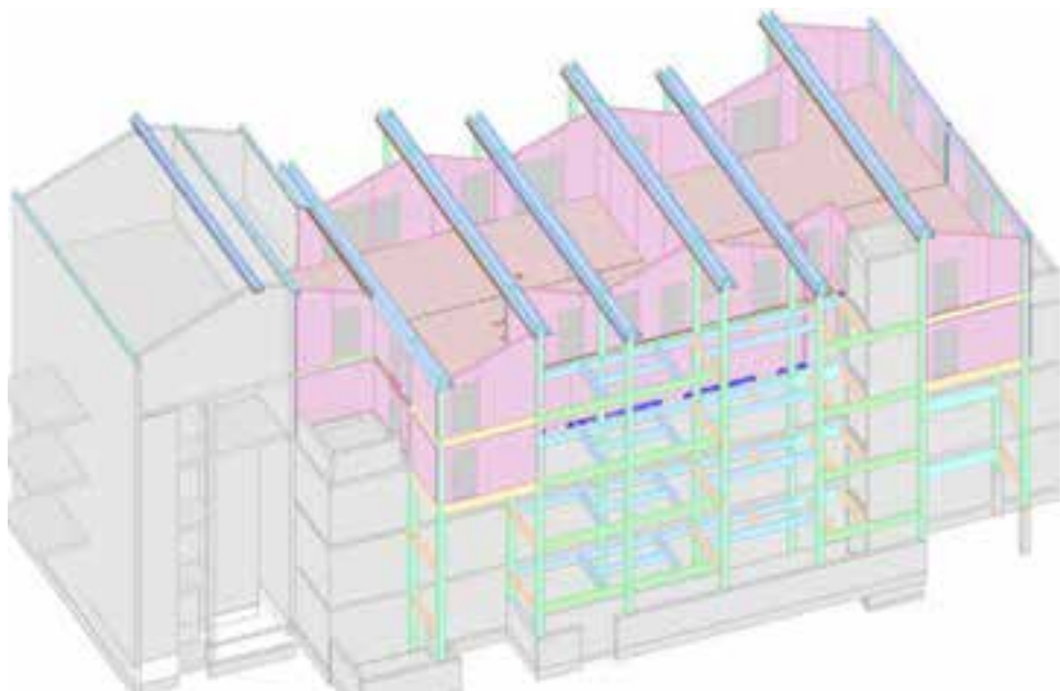
Surélévation du bâtiment B d'un niveau – éléments de façades en ossature bois préfabriqués © Toitures Montiliennes
