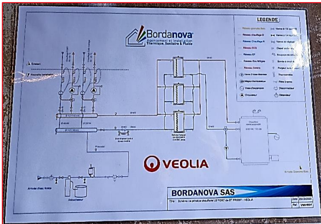
Schéma de principe de l'installation
